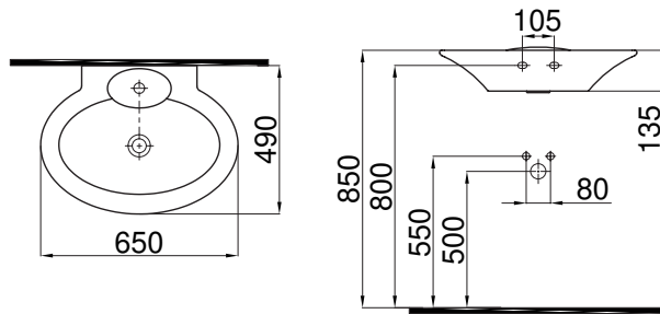
2901-0505 | Rena Tezgah Üstü Lavabo (49x65) Rena Countertop Washbasin
